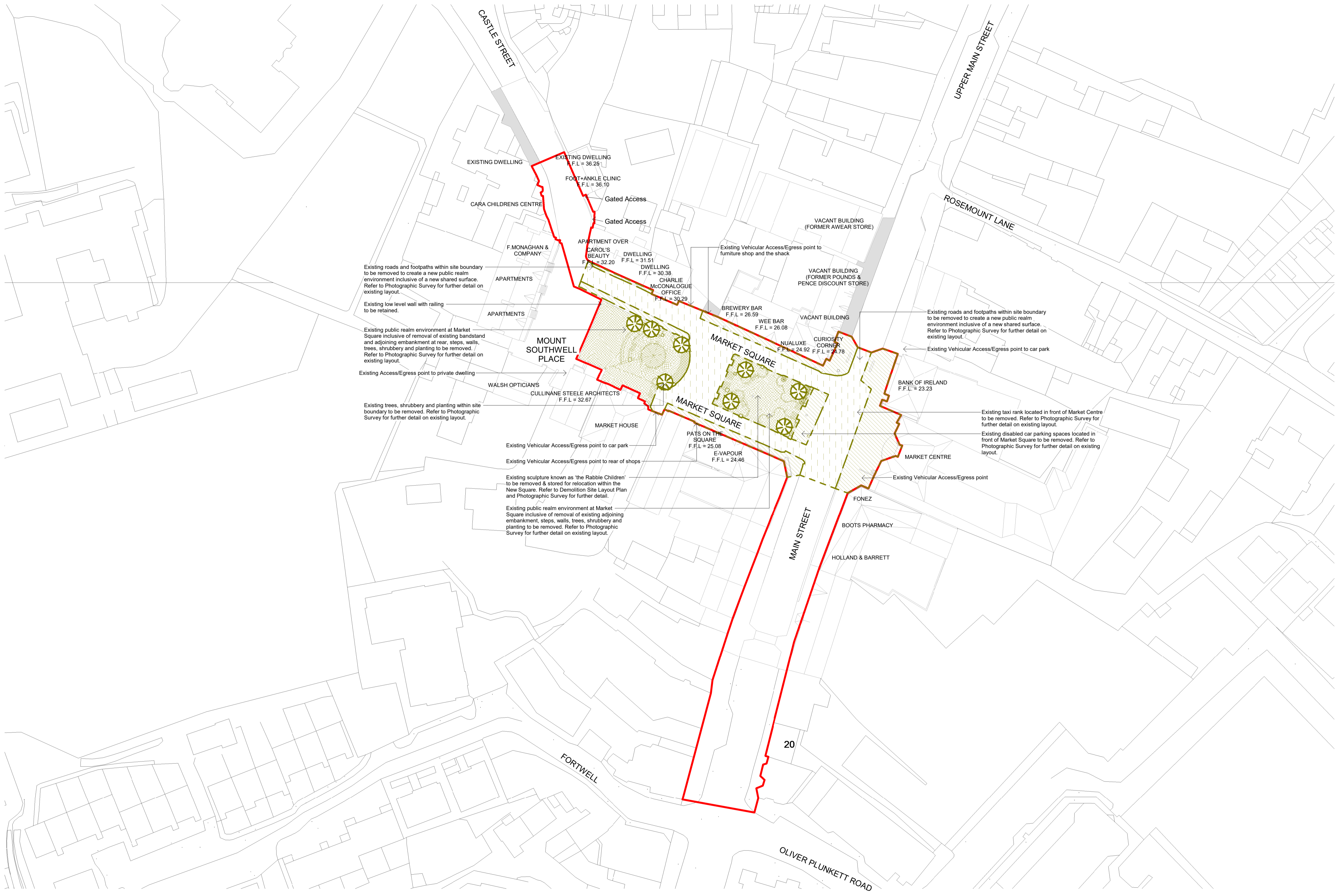
Demolition Site Layout Plan 1 : 500
